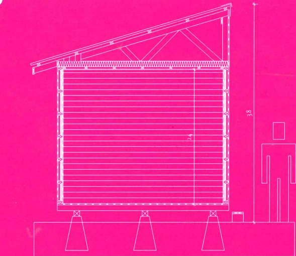
Corte constructivo Baulicher Querschnitt Constructive section
