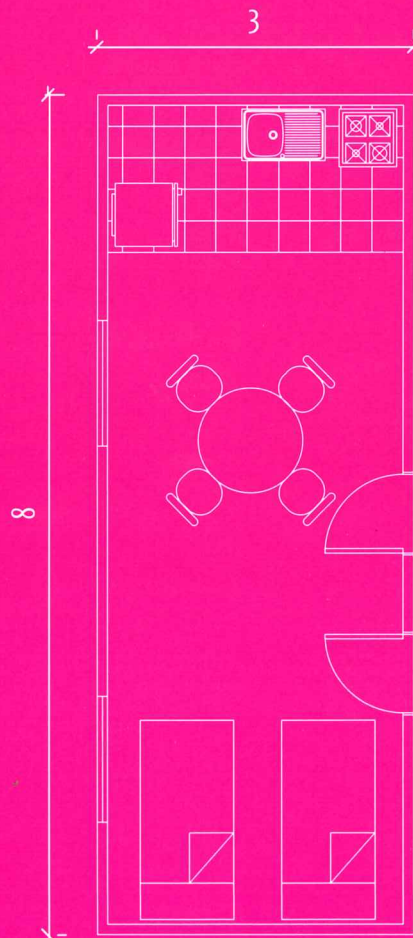
Planta de arquitectura Grundriss Master architectural plan
