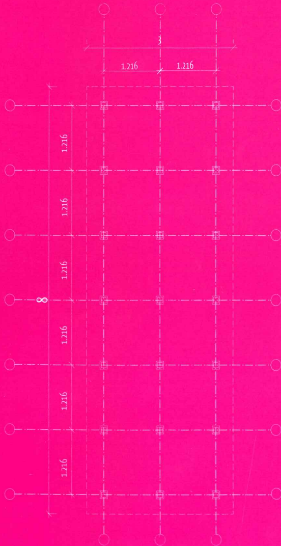
Planta de estructuras pilotes Stelzenstruktur Pile structure plan
